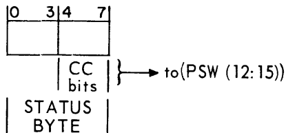
Figure 1-9. Status Byte Format
