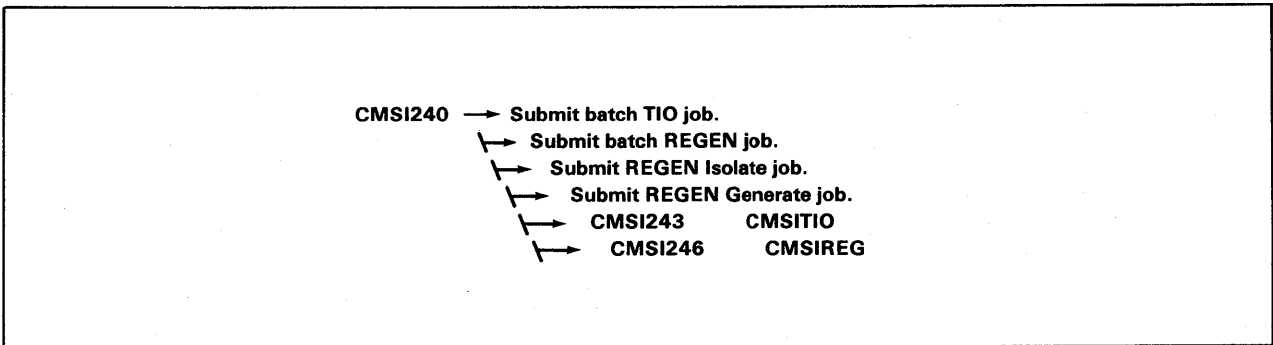
Figure 1-23. TIO/REGEN Interface Flowchart
