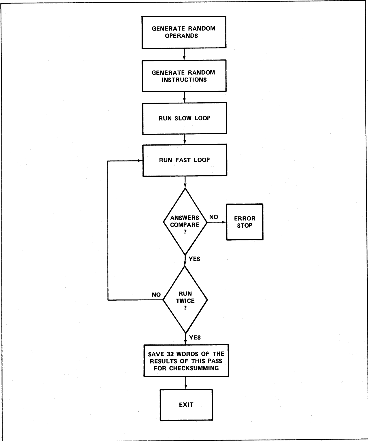
Figure 4-3. FST Flowchart
