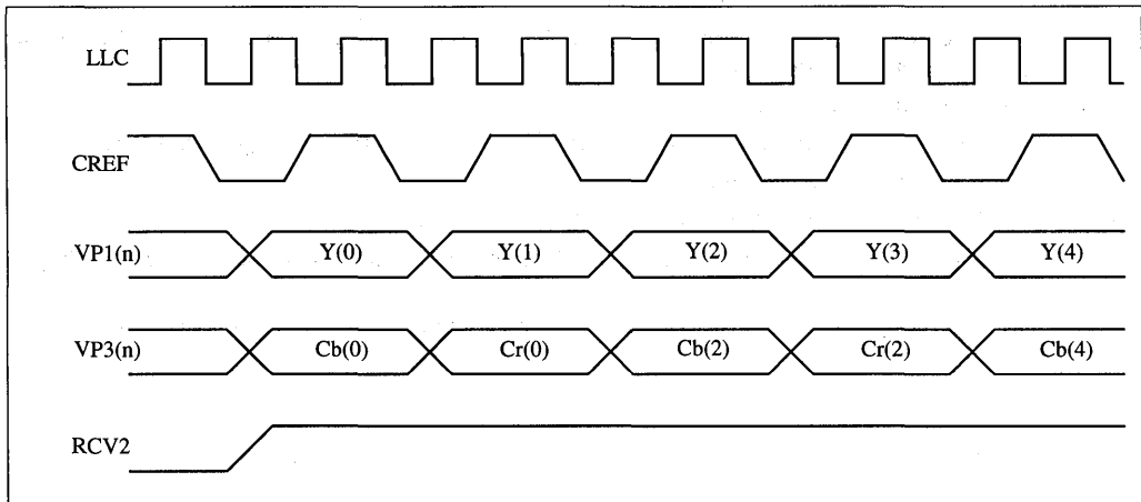
Fig. 12: Dig.TV - Timing
