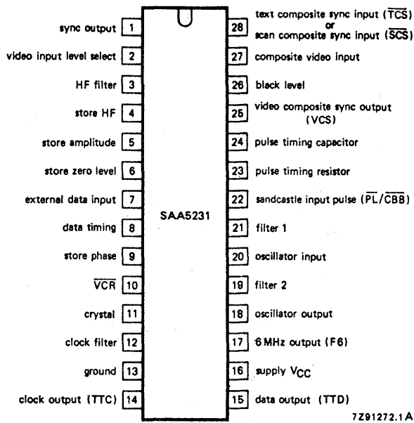
Fig. 2 Pinning diagram.
