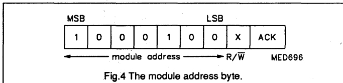
Fig.4 The module address byte.
