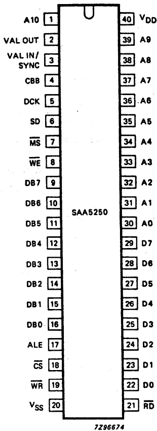
Fig. 2 Pinning diagram.
